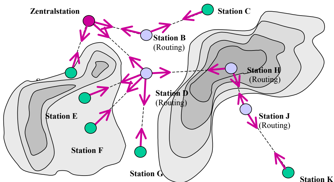
Struktur eines Datenfunknetzes zur automatischen Erfassung von Messwerten für das Lastmanagement in einem Gebiet mit einer Ausdehnung von ca. 500 km 2 und deren Übertragung zu einer Zentralstation unter Berücksichtigung der Umgebungsbedingungen (Zeitschlitzverfahren)
